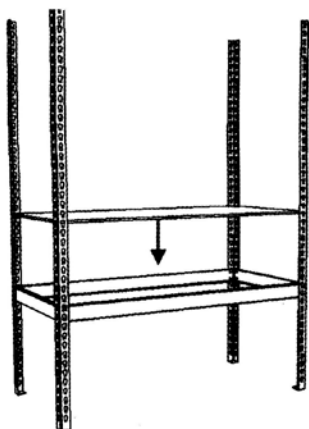
РИС. 4. Укладка фанерного настила
